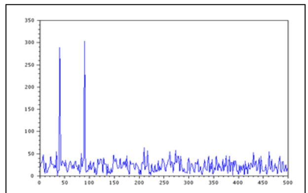
Figure 9 : TFD d'un signal composite à 40Hz et 90Hz
