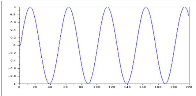
Figure 2 : Un centième de seconde d'un son sinusoïdal à 440 Hz
